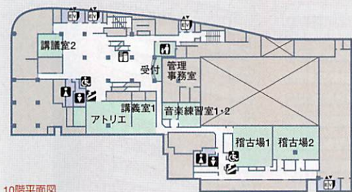
10階平面図
